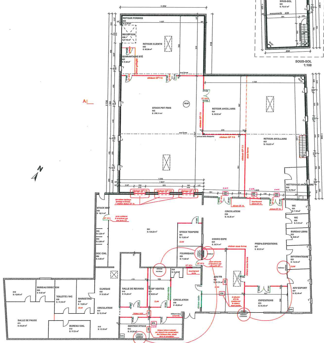
REZ-DE-CHAUSSEE 1:100
