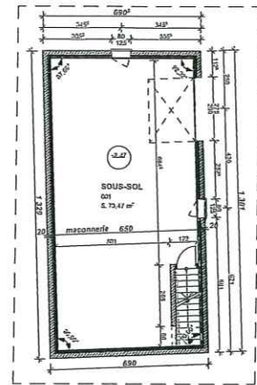
SOUS-SOL 1:100
