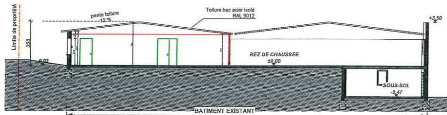
COUPE A 1:100
